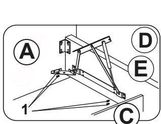
Крепление подъемного механизма к боковым царгам. Для кроватей с размером спинки 80 - крепление на 2 винта, для кроватей с размером спинки 90 - крепление на 4 винта
