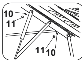
Крепление подъемного механизма к ортопедическому основанию (внутренняя сторона) (газлифт крепится к подъемному механизму цилиндром вверх как на схеме)
